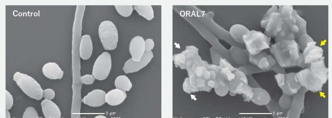
オーラルセブンで処理した C. albicans は細胞表面に皺が認められる（白矢印）。また一部破損している細胞も認められる（黄矢印）。
